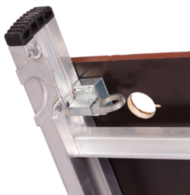
ΜΗΧΑΝΙΣΜΟΣ ΠΛΑΤΦΟΡΜΑΣ ΜΕ ΠΟΡΤΑ
